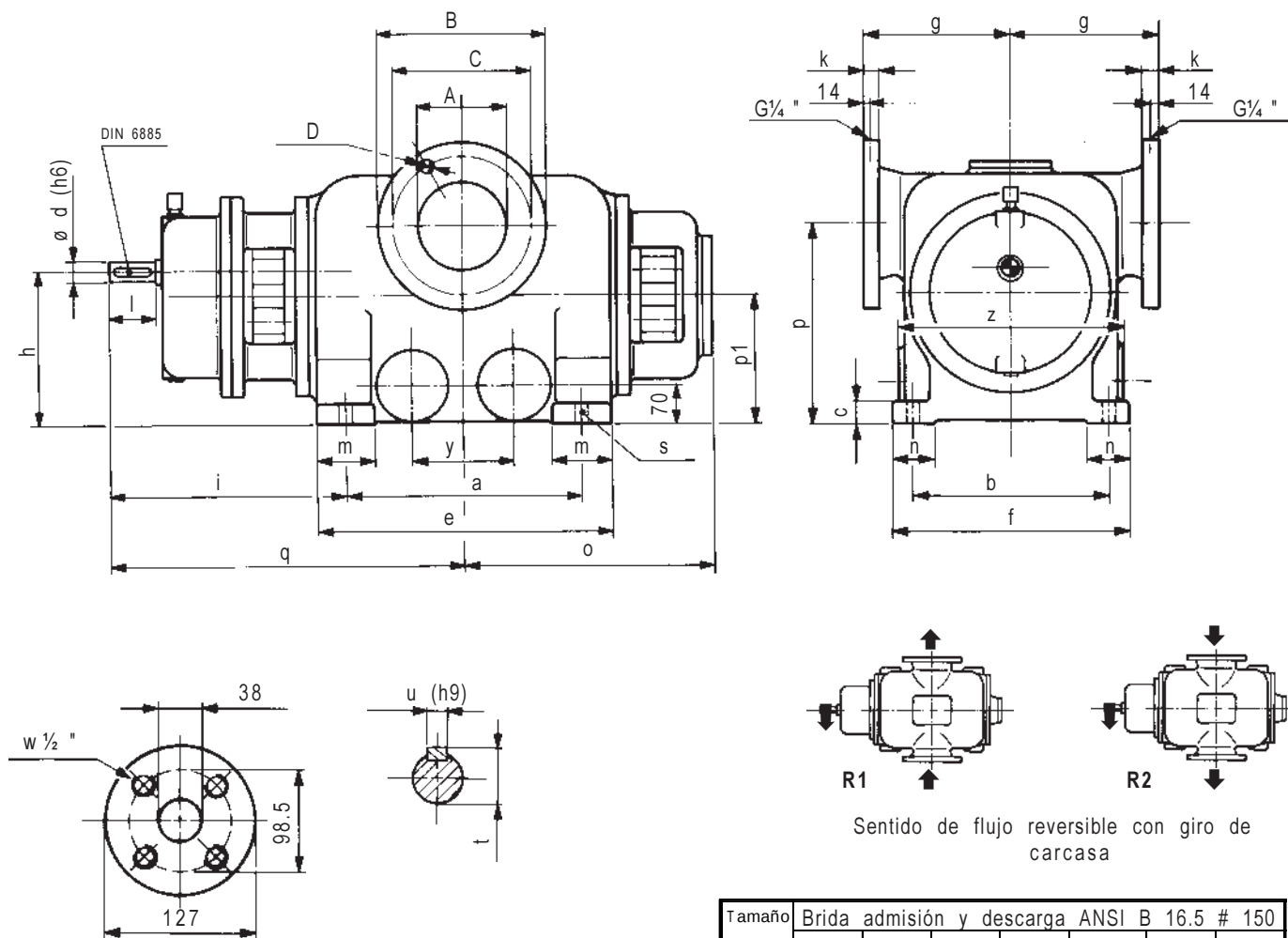
Brida calefacción 1/2 " ANSI B 16.5 # 150
